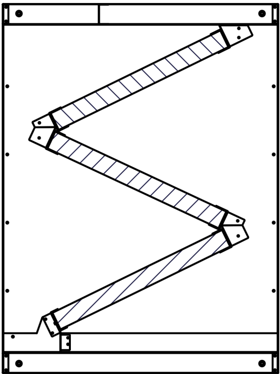
F-F ( 1 : 10 )
